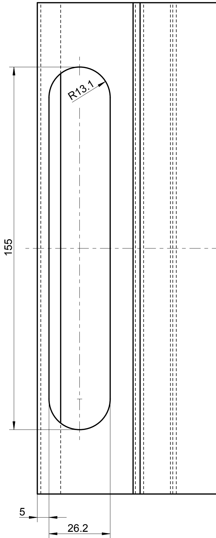
Fräsbild Stahlzarge Rahmen
