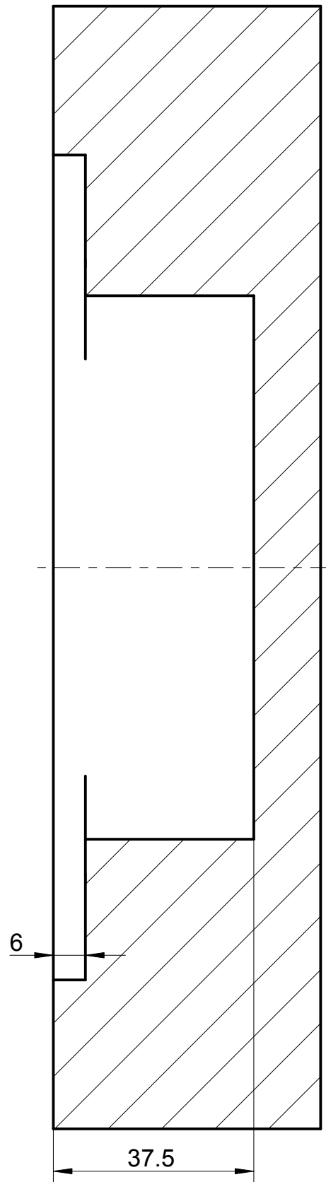
Fräsbild Flügel
