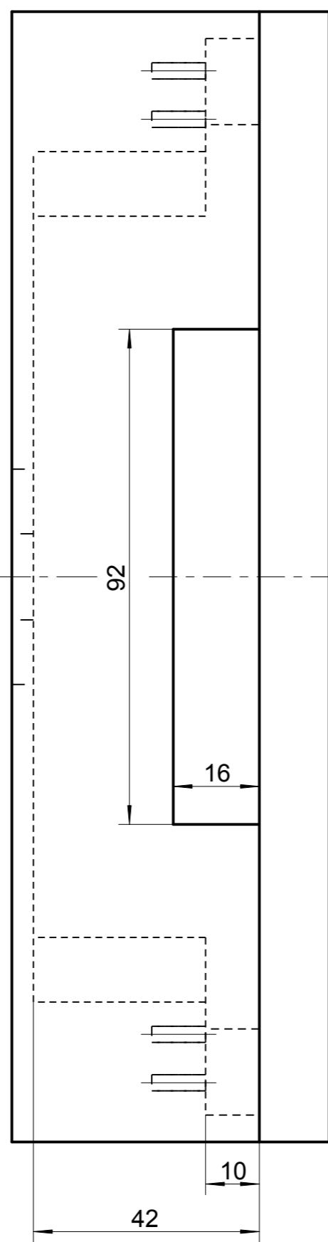
Fräsbild Blockzarge Rahmen
