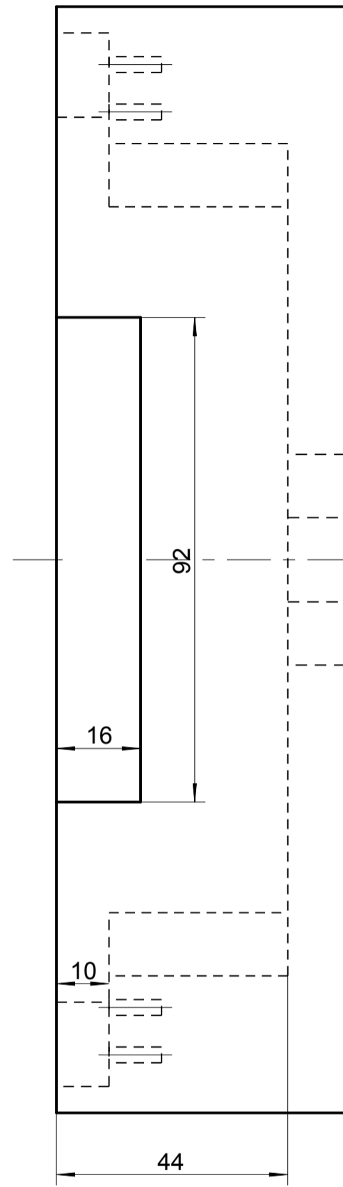
Fräsbild Flügel
