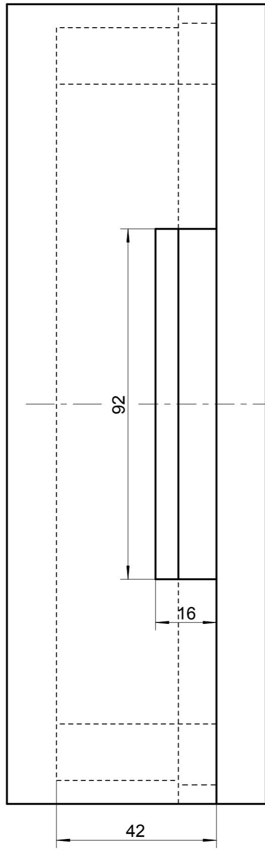
Fräsbild Futterzarge Rahmen
