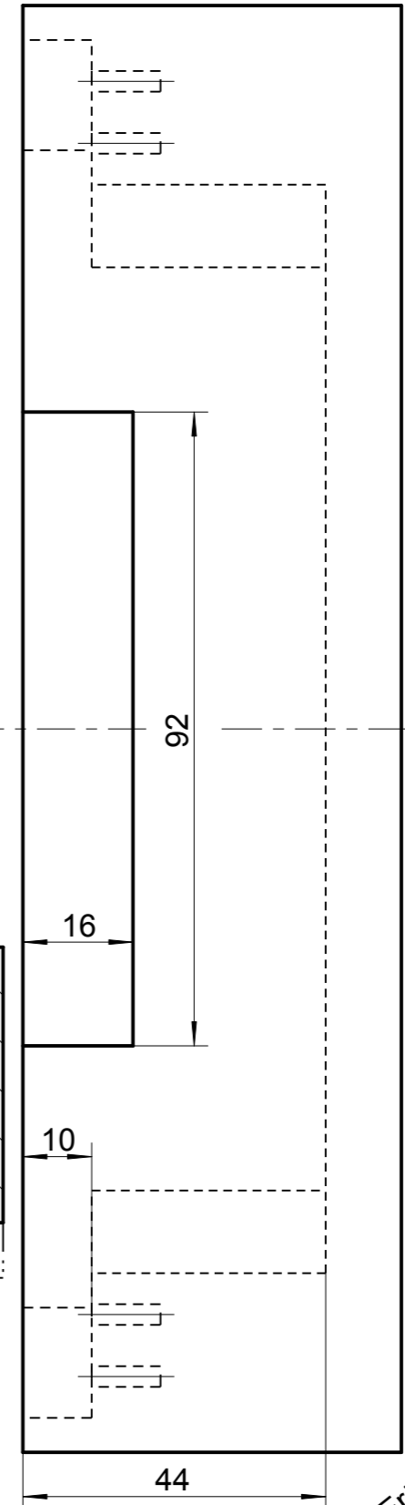
Fräsbild Flügel
