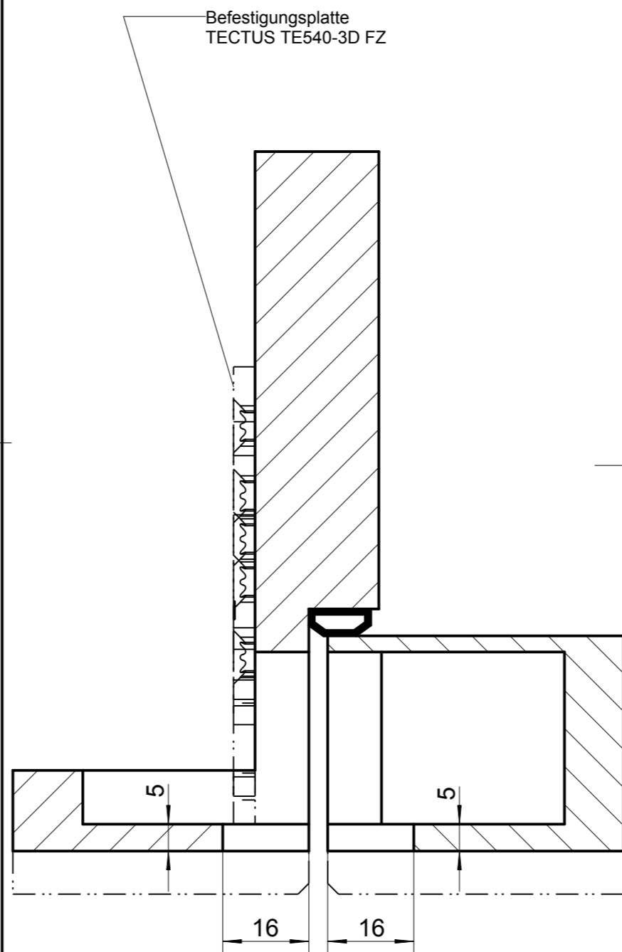
Fräsbild Flügel
