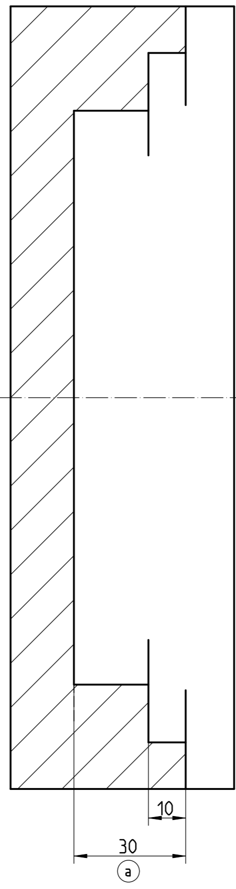
Fräsbild Rahmen Blockzarge
