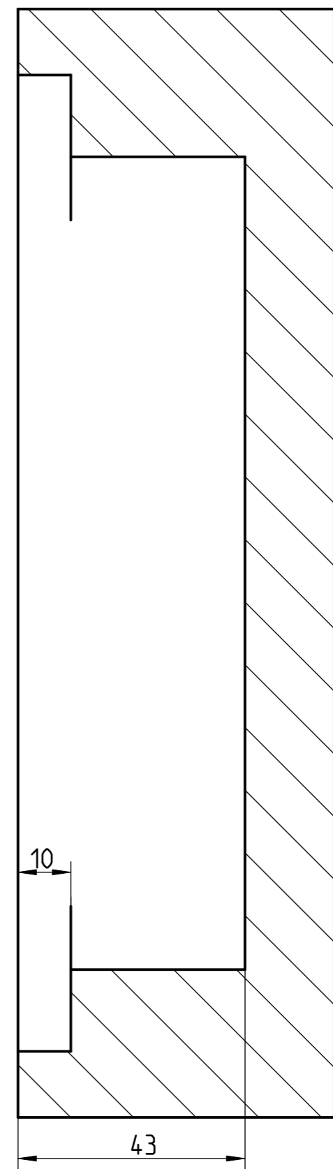
Fräsbild Flügel
