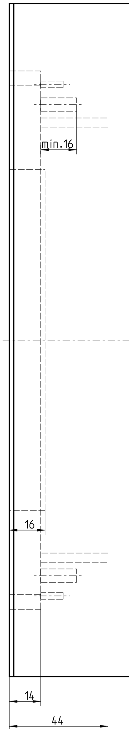
Fräsbild Flügel m. Aufdoppelung
